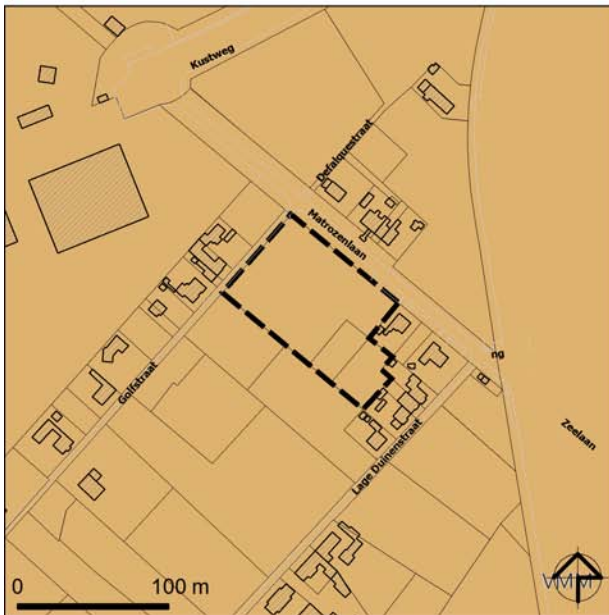
WATERTOETS GRONDWATERSTROMINGSGEVOELIGE GEBIEDEN bron: VMM
