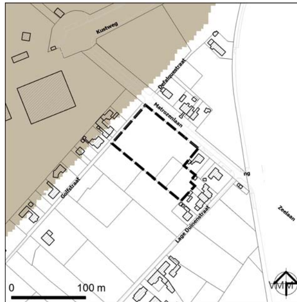
WATERTOETS INFILTRATIEGEVOELIGHEID bron: VMM
