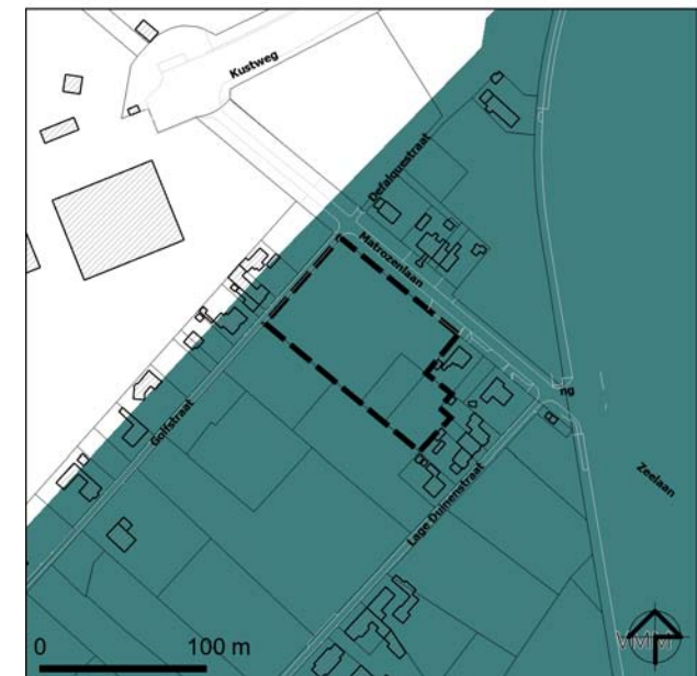
WATERTOETS OVERSTROMINGSGEVOELIGHEID bron: VMM
